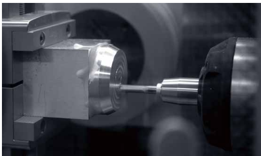
铣削
